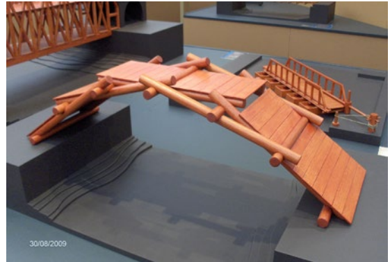
Kleine zelfdragende brug
